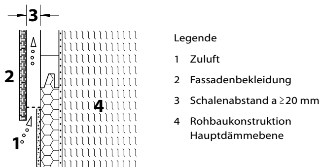
Abb. 53: Die Bekleidung wird auf einer Traglattung befestigt. Die Ebene der Traglattung bildet die notwendige Luftschicht.
