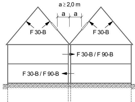
Abb. 30: Dächer giebelständiger Gebäude in den Gebäudeklassen 1-3. Der erforderliche Abstand der Dachflächenfenster (DFF) von der Gebäudeabschlusswand beträgt mindestens 2 m.
