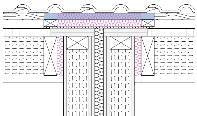
Abb. 27: Dachanschluss einer Gebäudeabschlusswand.
