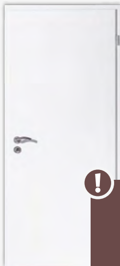
Schallschutz-Türblatt (SST) und Zarge SR-Kante Decora (CPL) Brillant Weiss Schallschutz (RWP 32 dB) Prüfklima „b + c“ inkl. Bodendichtung 3-tlg. Bänder, vern., PZ-vorgerichtet
